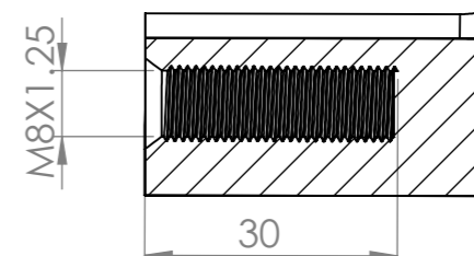
SECTION D-D SCALE 1:1
